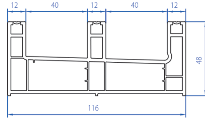
3T Sliding Frame 3104-3102
