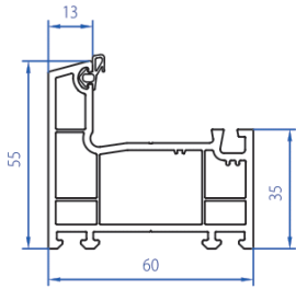
Casement Frame 2101-1101
