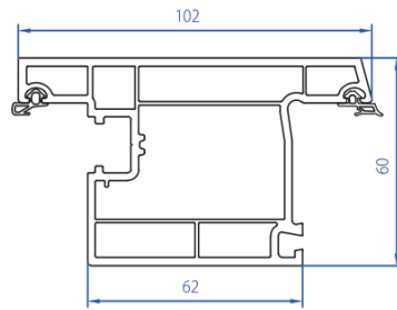
Outward Door Sash 2103-1102
