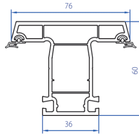
T-Mullion 2102-1101
