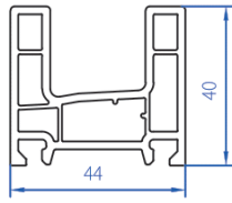
2T Frame 4104-3101
