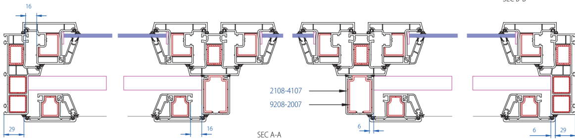
SEC A-A
