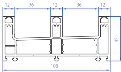
3T Sliding Frame 2104-3102
