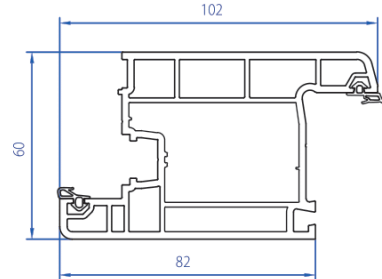
Inward Door Sash 2103-1104
