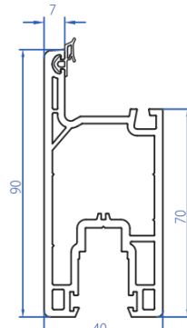
Sliding Door sash 2105-1103
