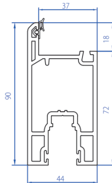
Sliding Door sash 3105-1103
