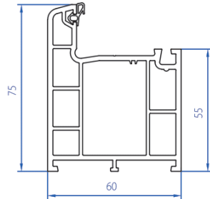
Door Frame 2101-1103
